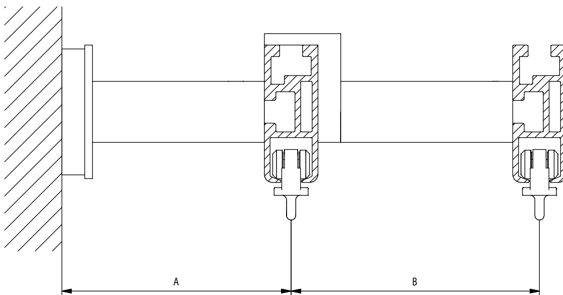
Installazione a parete sistema doppio
