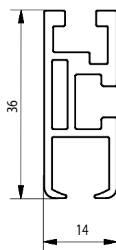
Profilo D21020 - scala 1:1
