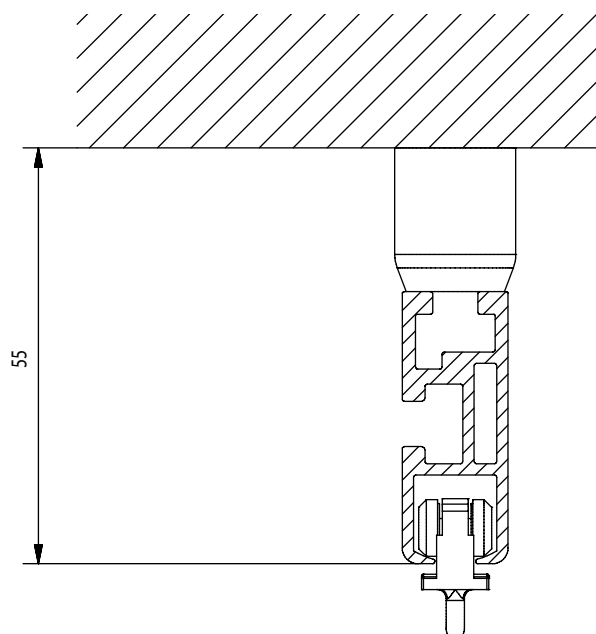
Installazione a soffitto
