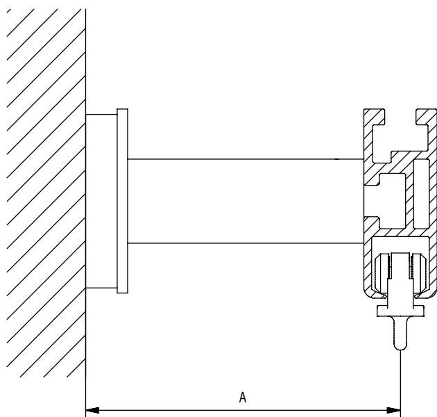
Installazione a parete sistema singolo
